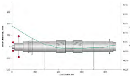
Biegeschwingsform einer Ritzelwelle
